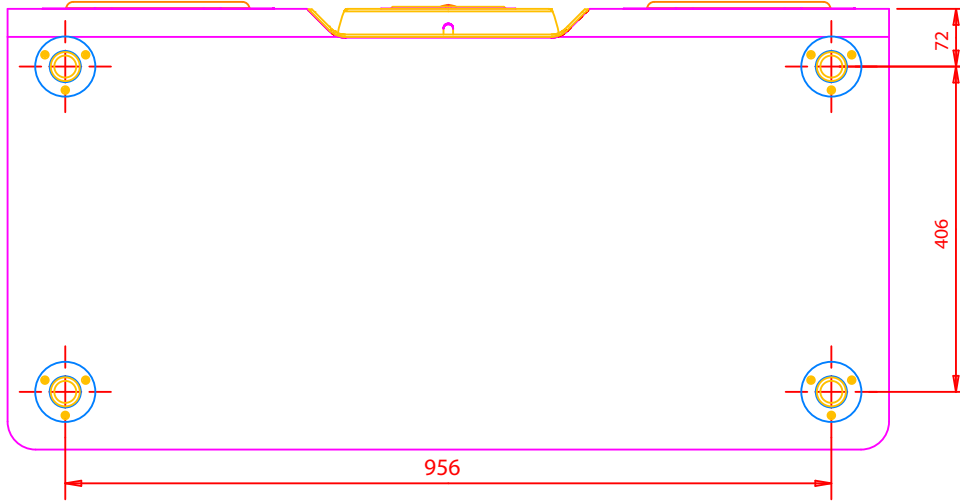
4-BOTTOM
